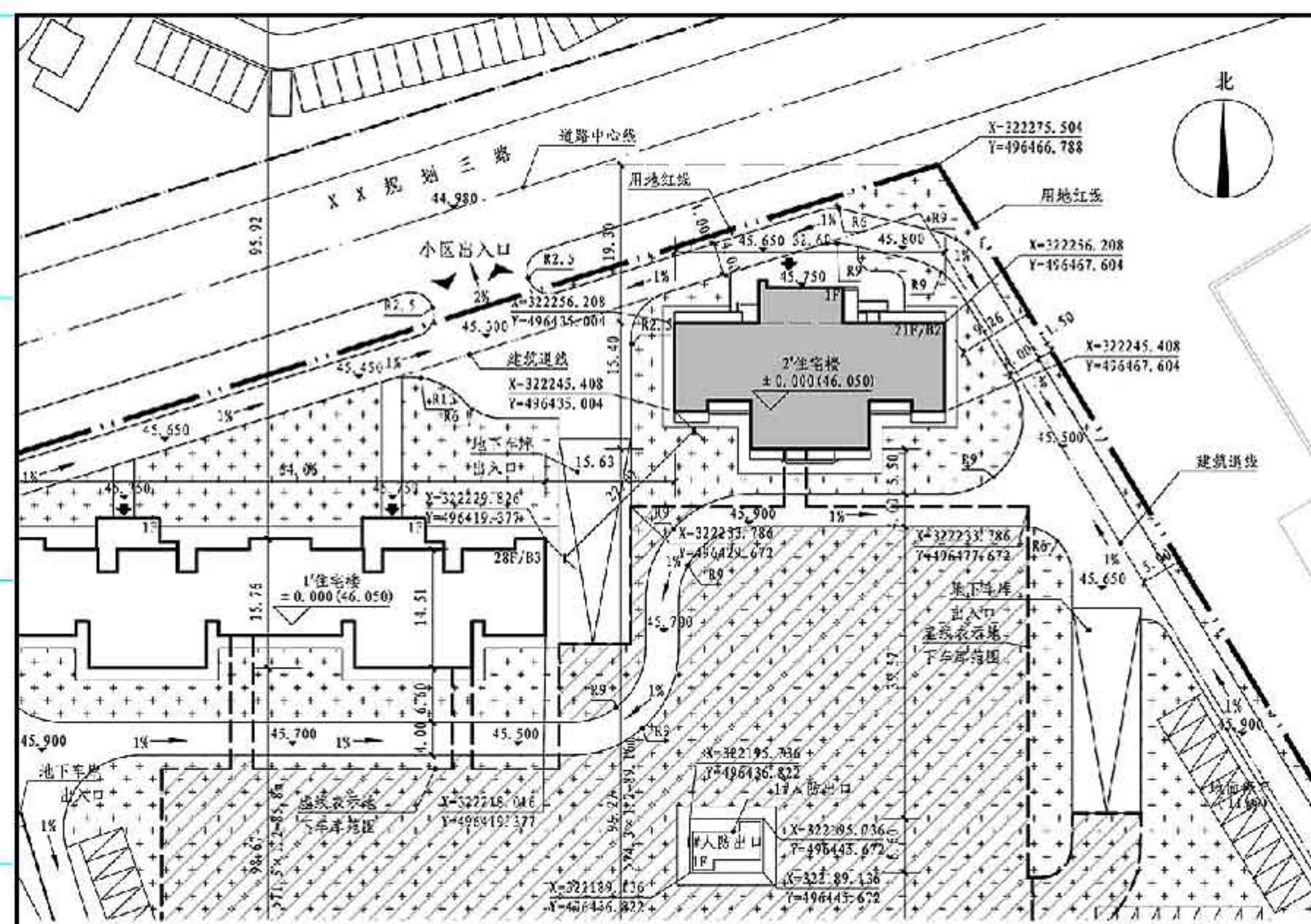
总平面图 1:500
