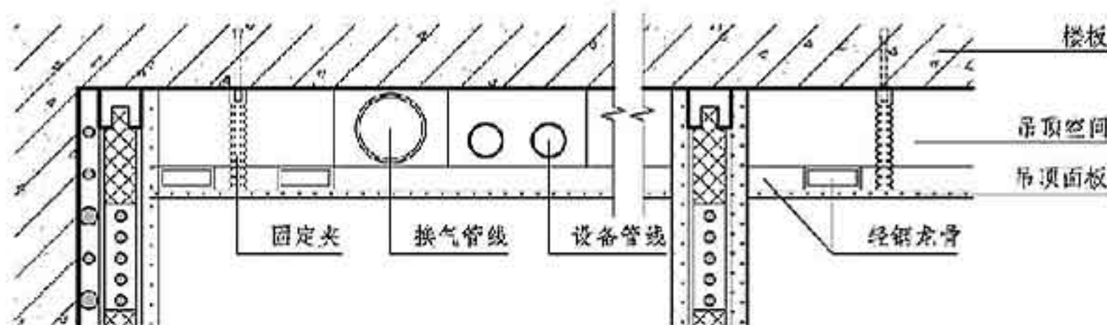
图5 双层顶板示意图
