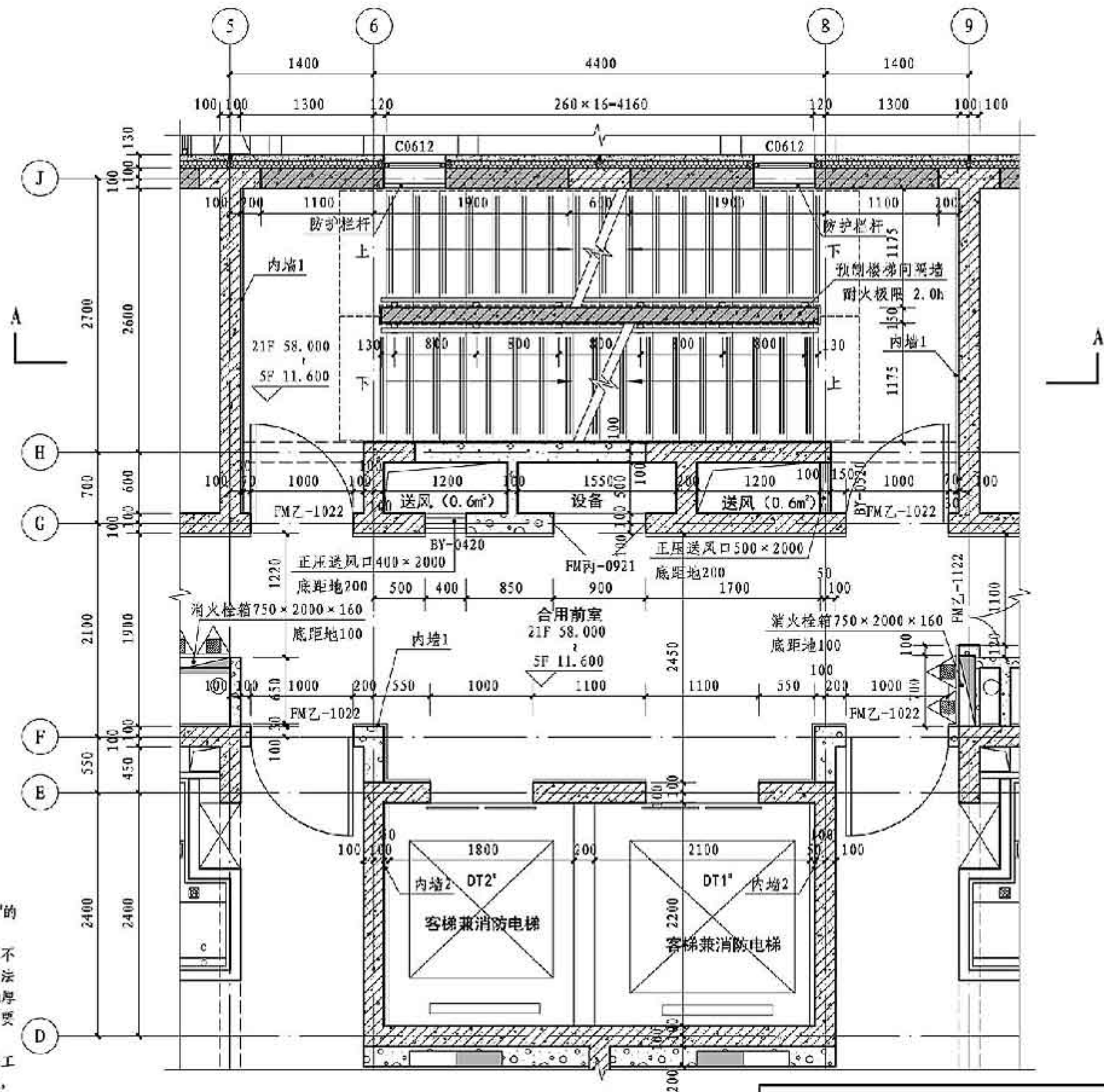
楼、电梯平面详图 1:50
