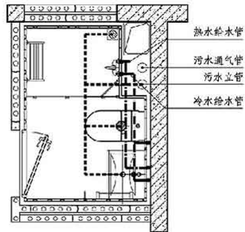
给排水管线示意图
