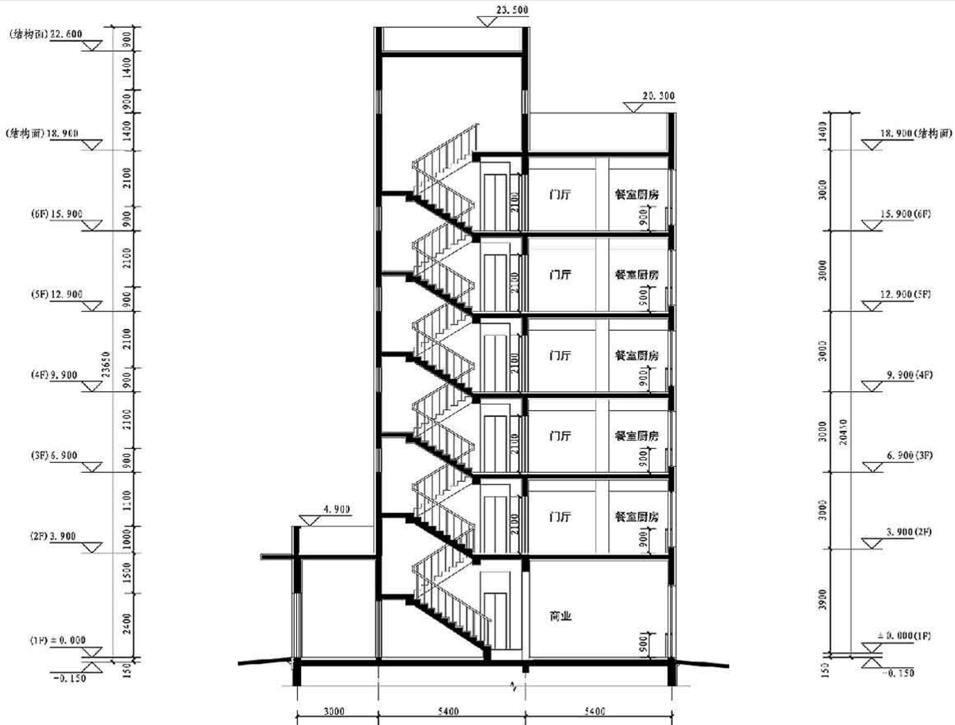
1-1剖面图
