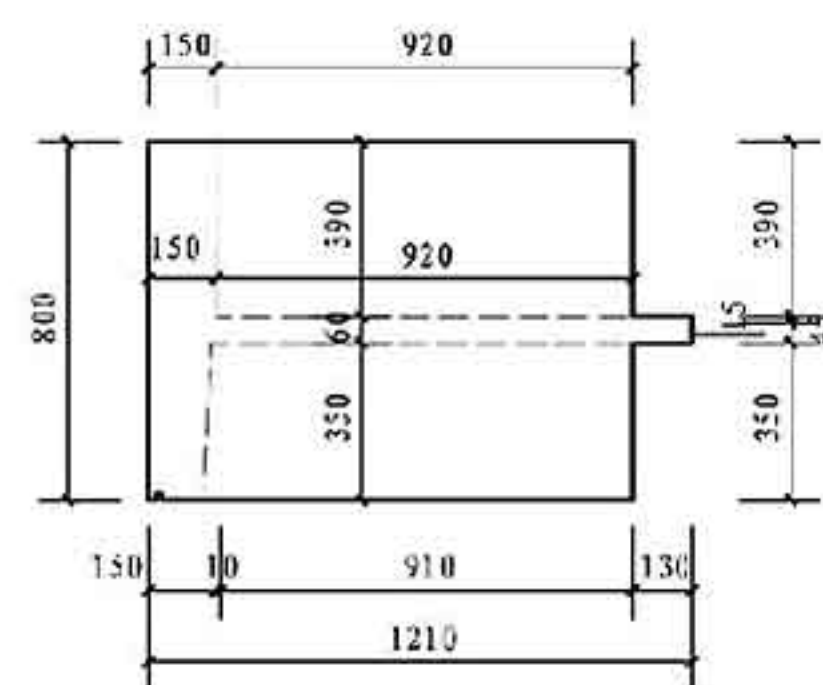
右视图 1:50
