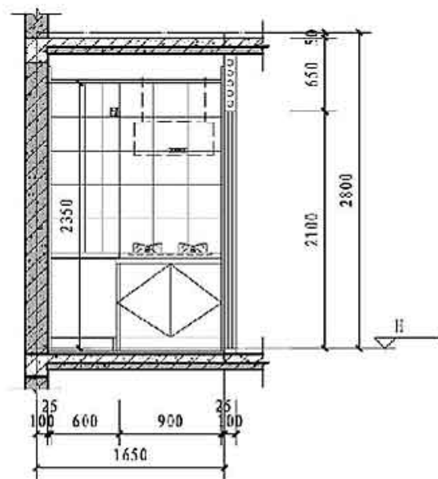
D-D剖面图 1:50
