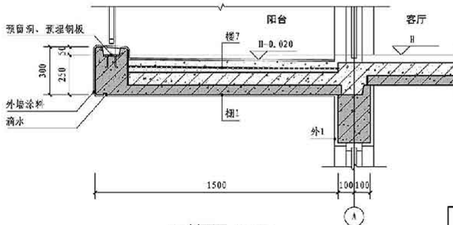
B-B剖面图 1:20
