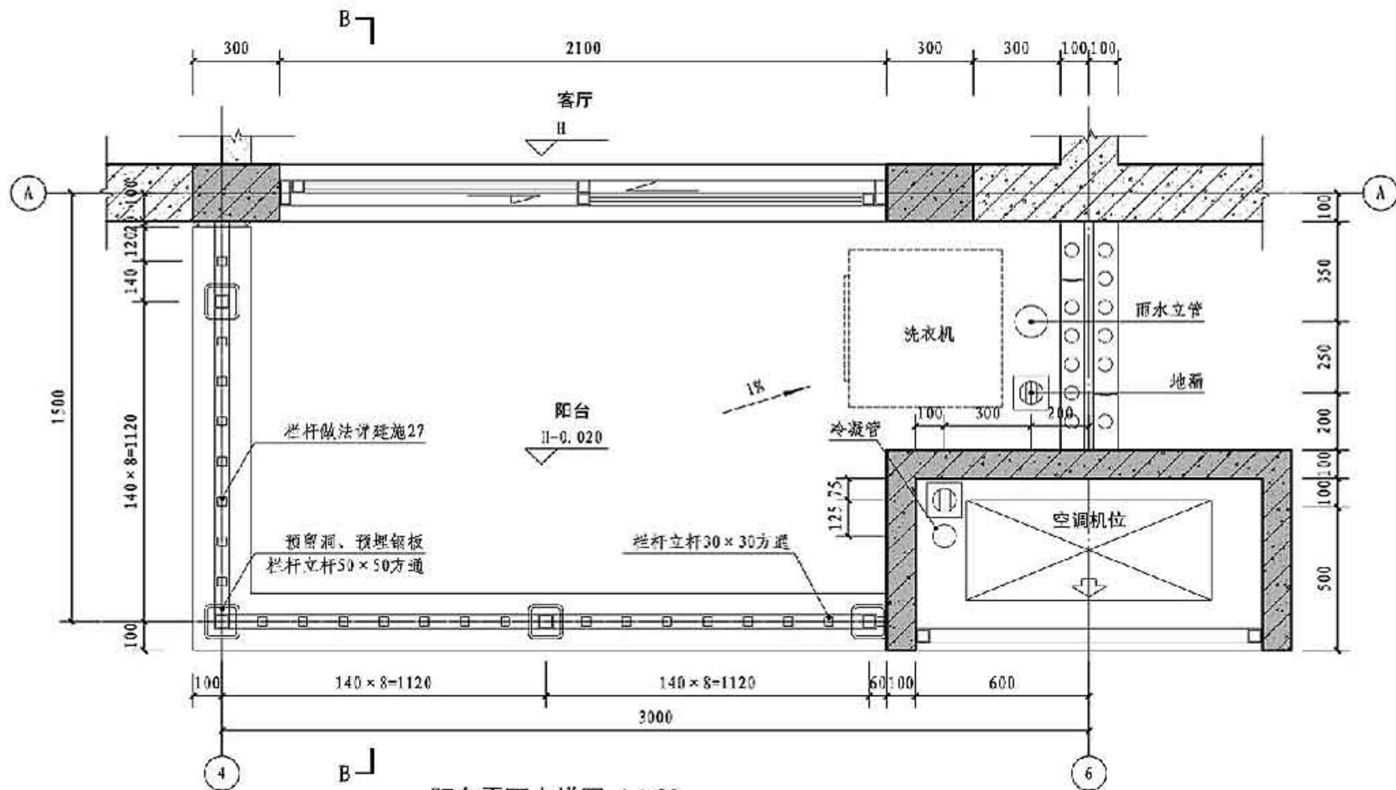
阳台平面大样图 1:20
