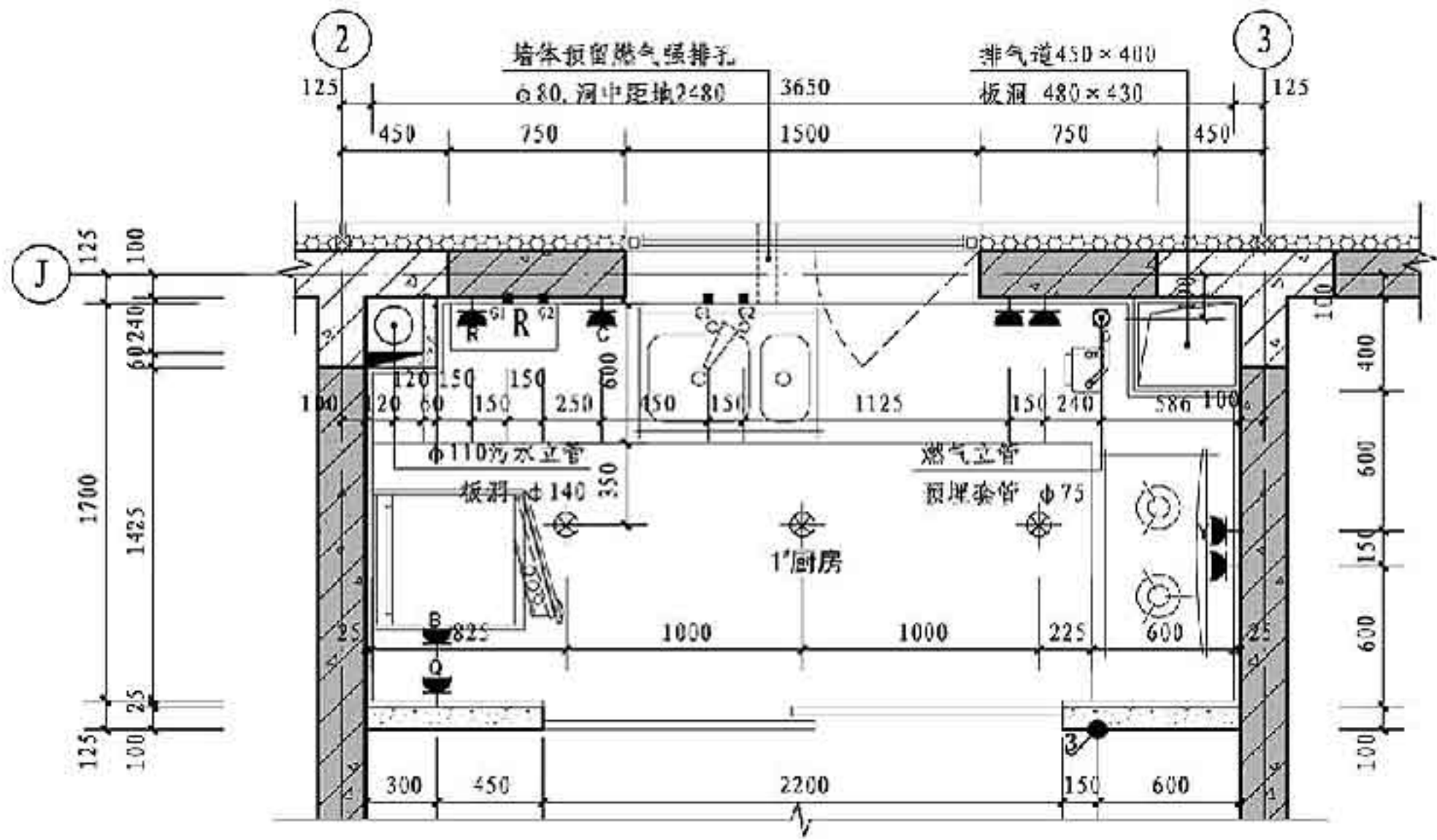
1 楼 厨房大样图 1:30
