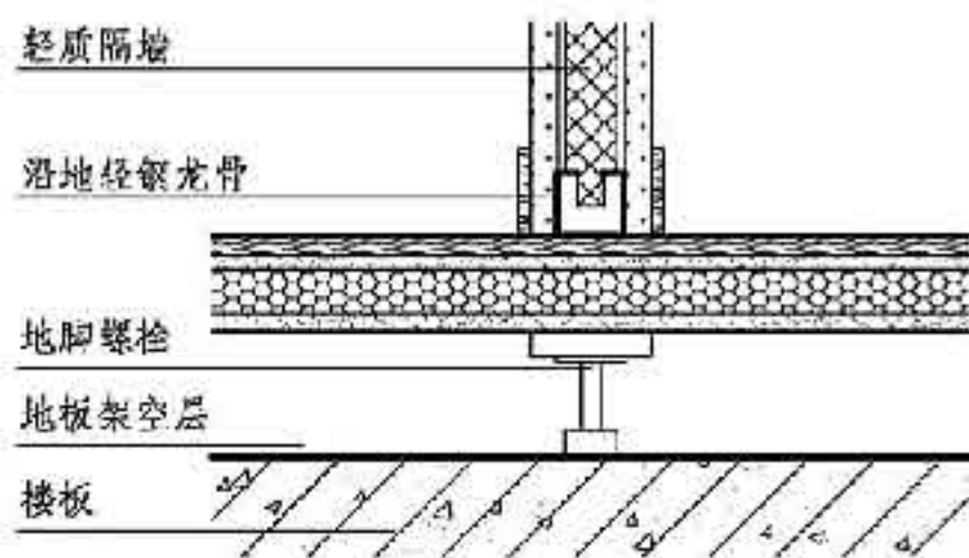
图2 SI住宅体系地面优先施工示意图
