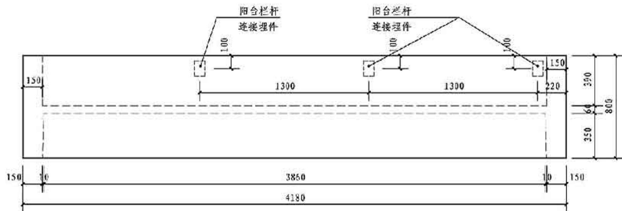
正视图 1:50
