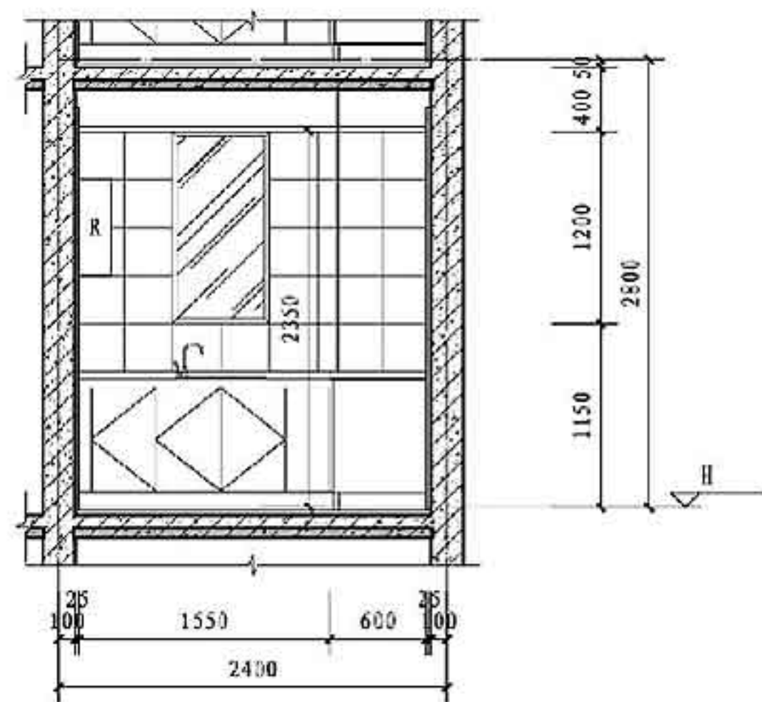
C-C剖面图 1:50
