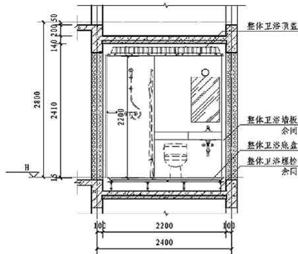
E-E剖面图 1:50
