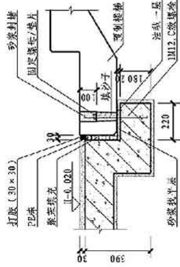
② 楼梯构件下端连接节点 1:10
