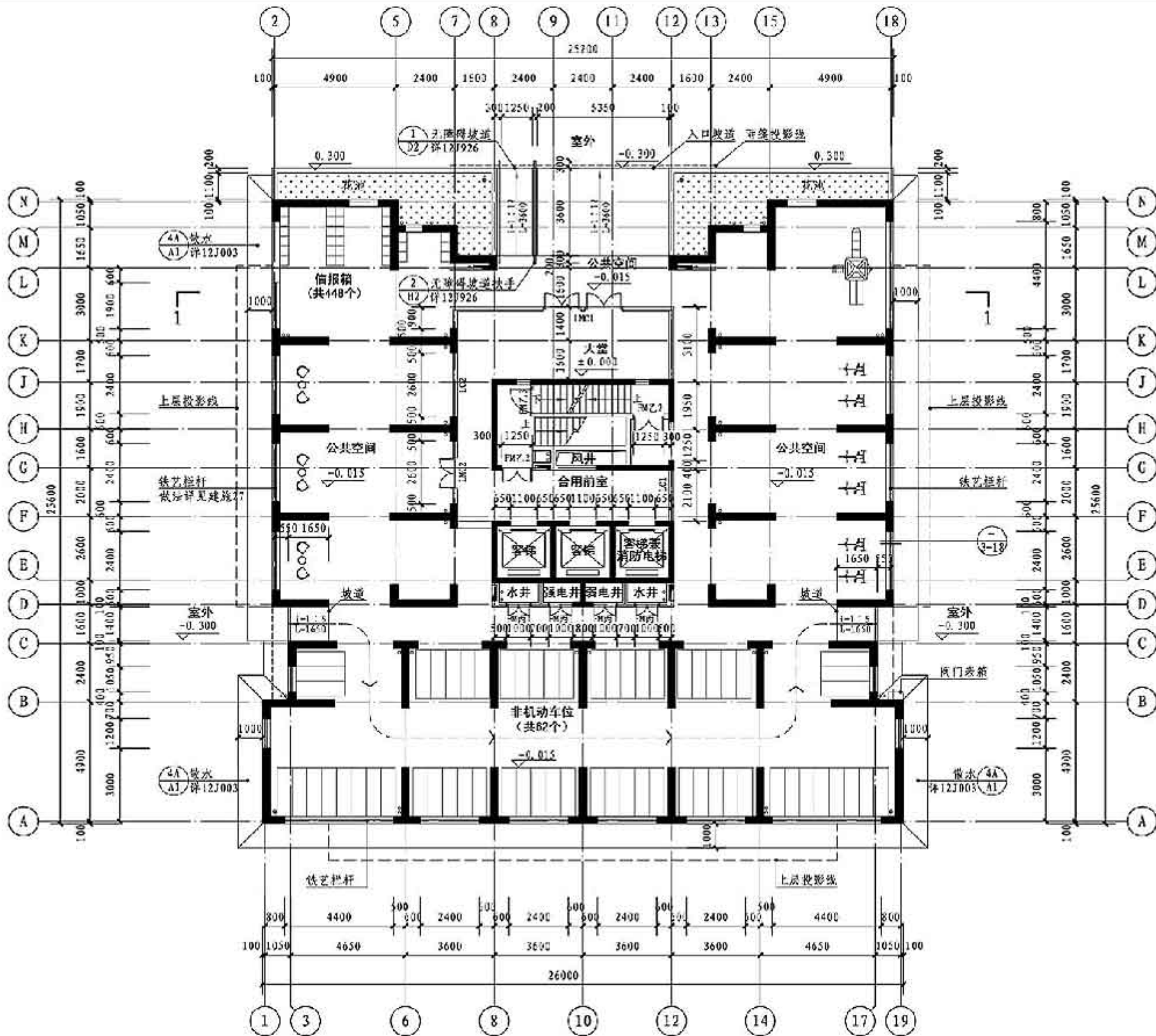
首层平面图 1:100
