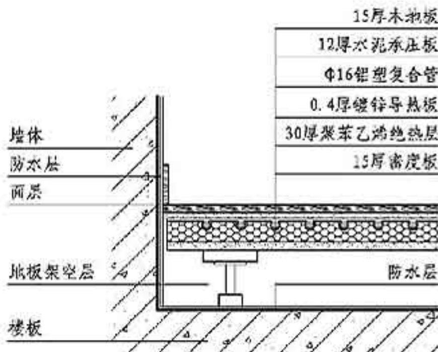
图4 干式地暖示意图（架空）
