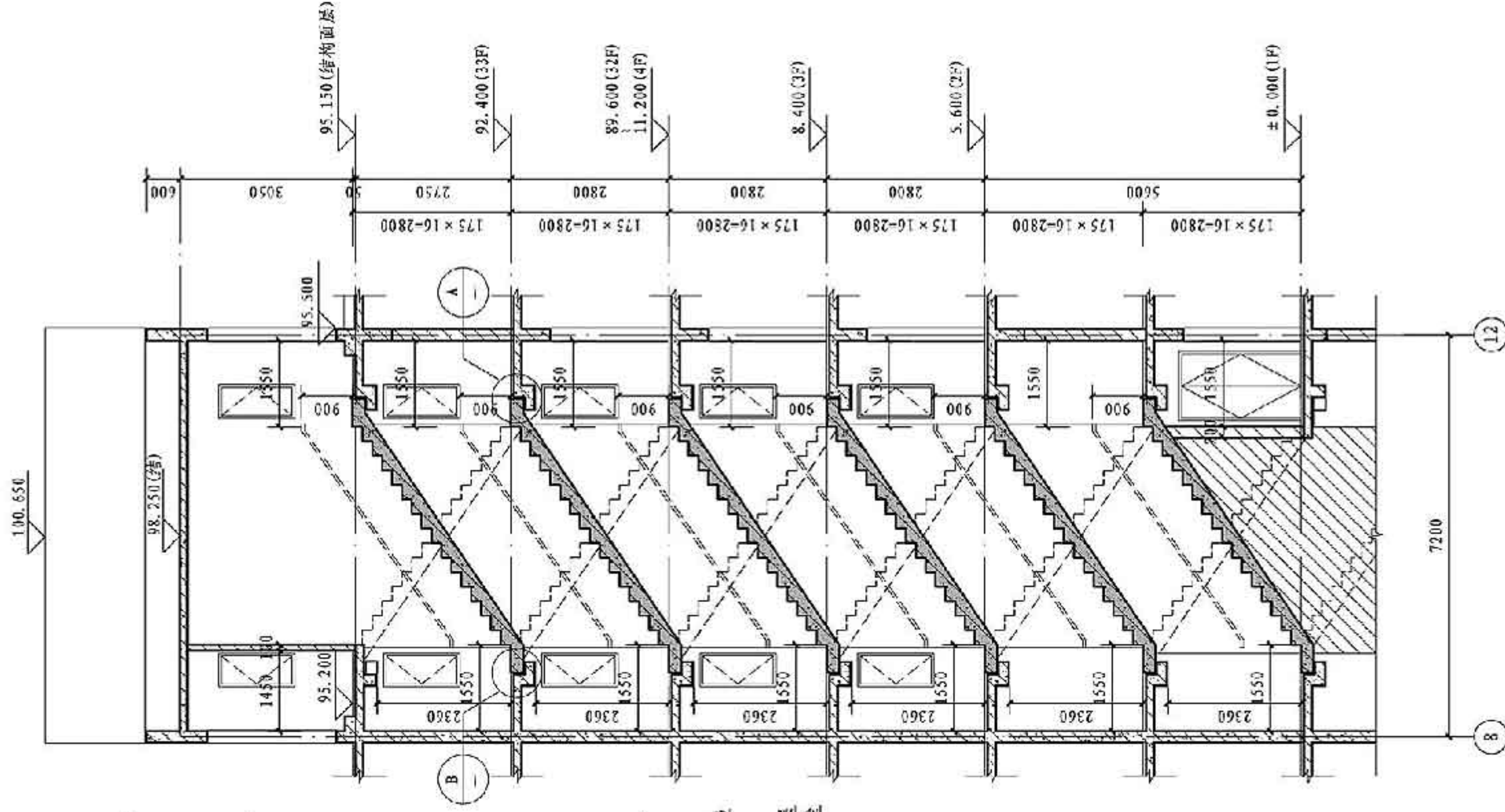
楼梯A-A剖面图 1:50
