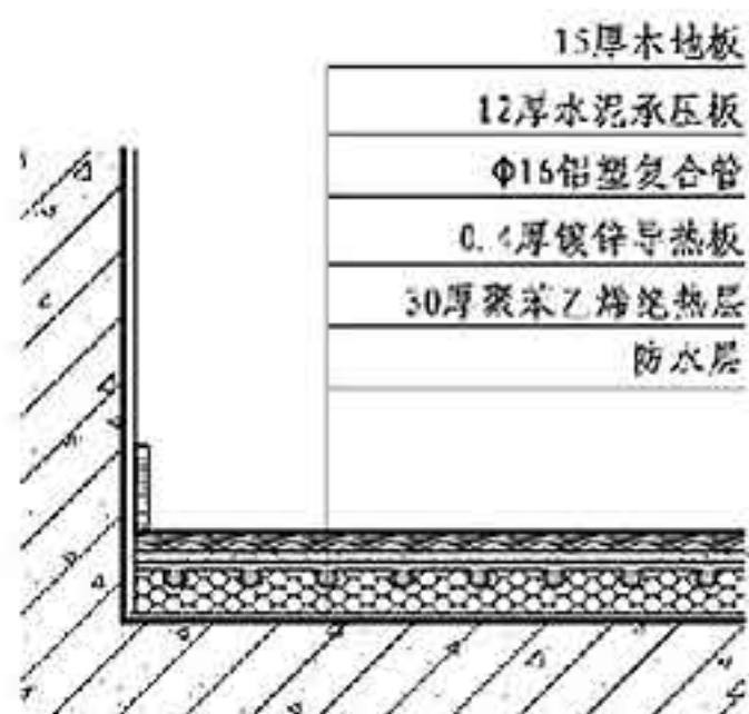
图3 干式地暖示意图（直铺）
