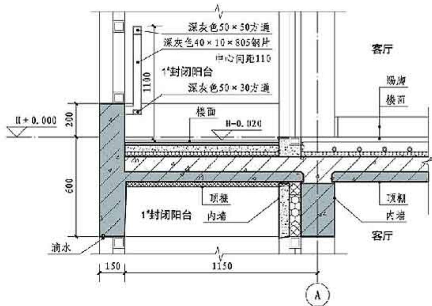
1 st 阳台B-B剖面图 1:20
