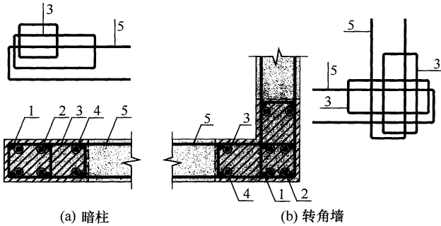
图 5.7.5-2 钢筋浆锚搭接连接长度范围
