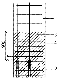
图 5.6.3-1 柱底箍筋加密区域构造示意
