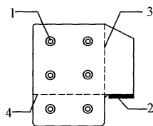
图 5.5.5-2 钢企口示意 1—栓钉；2—预埋件； 3—截面 A；4—截面 B
