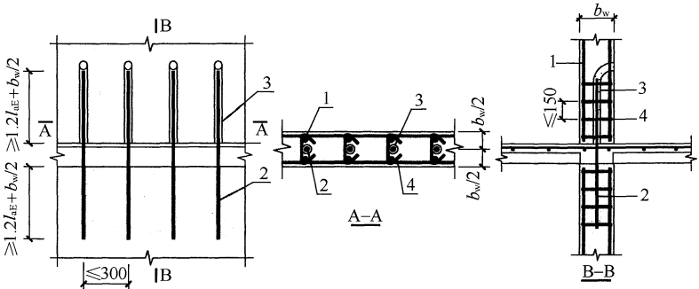
图 5.7.12-3 竖向分布钢筋单排浆锚搭接连接构造示意
