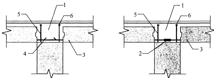
(a) 梁下部纵向受力钢筋锚固
