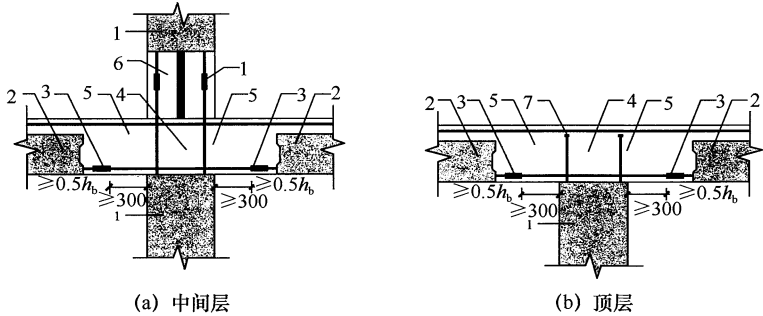
图 5.6.6-2 框架节点叠合梁底部水平钢筋在两侧梁端后浇段内采用挤压套筒连接示意 1—预制柱；2—叠合梁预制部分；3—挤压套筒；4—后浇区； 5—梁端后浇段；6—柱底后浇段；7—锚固板
