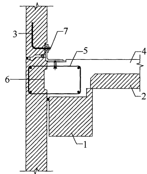
图 5.9.8 外挂墙板线支连接示意
