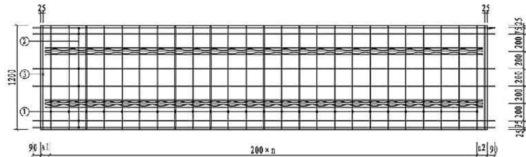
板配筋图
