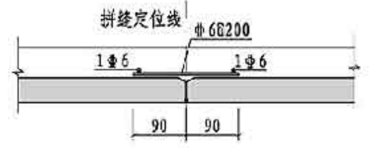
单向板拼缝构造大样
