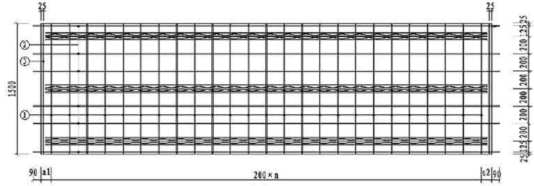
板配筋图
