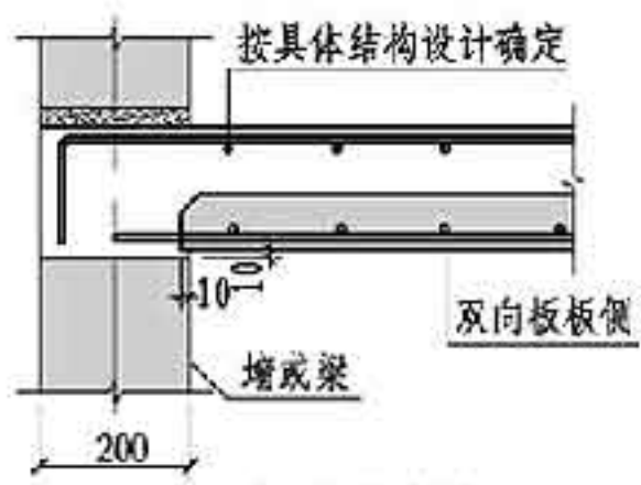
侧支座构造(三)
