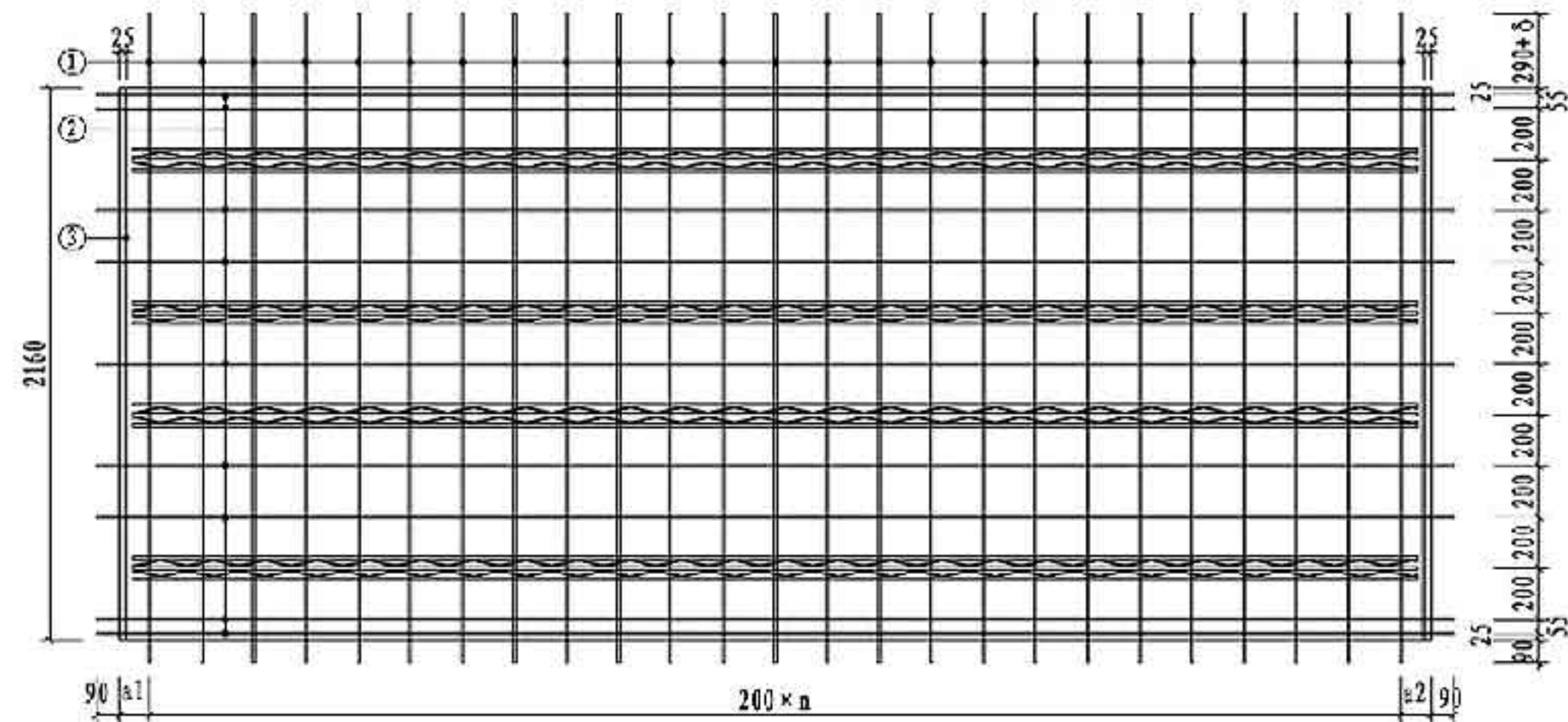
板配筋图
