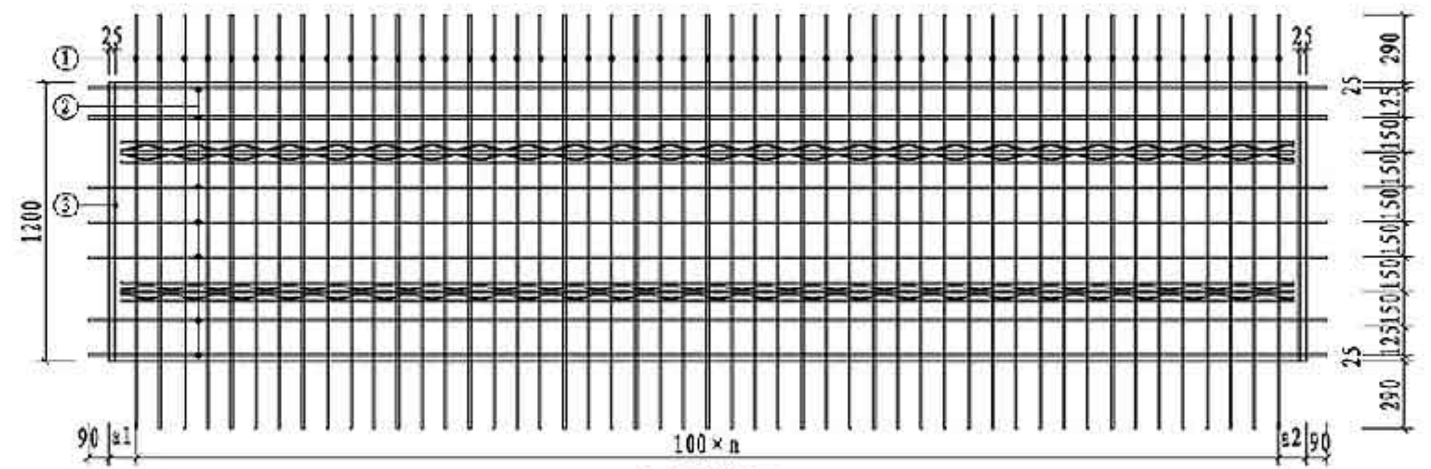
板配筋图
