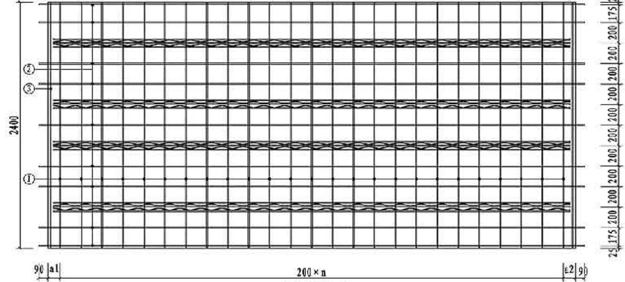
板配筋图
