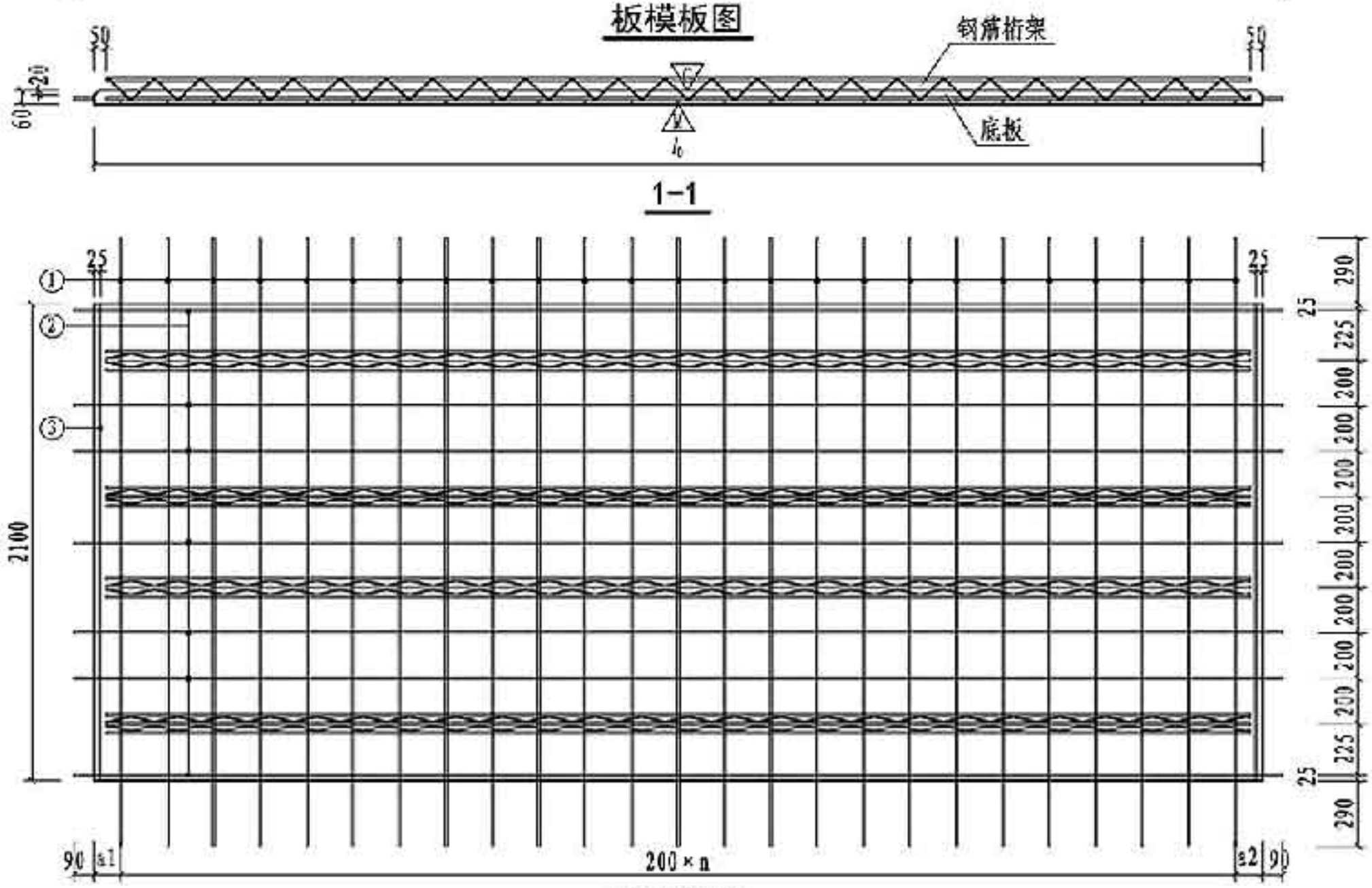
板配筋图
