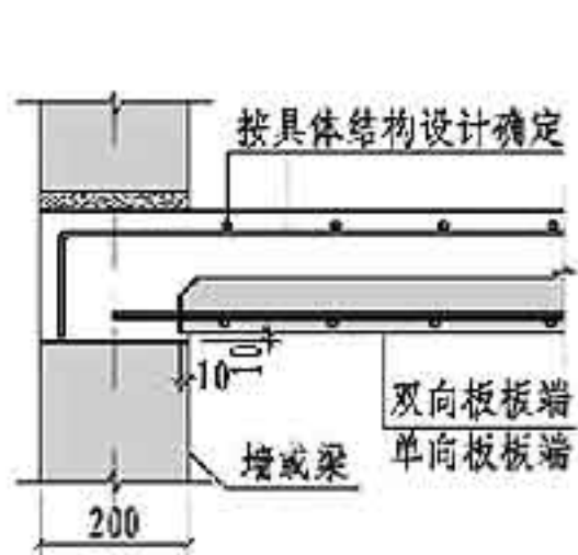
端支座构造
