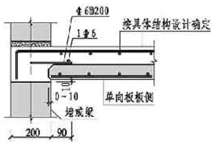
侧支座构造(一)
