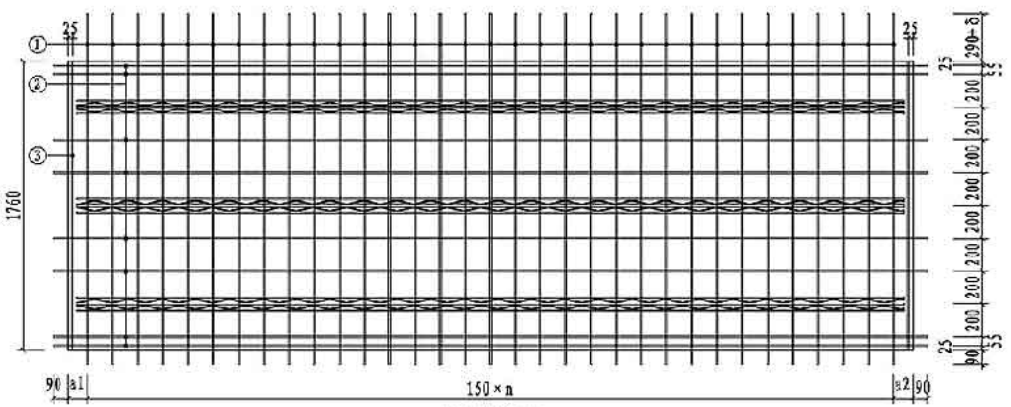
板配筋图
