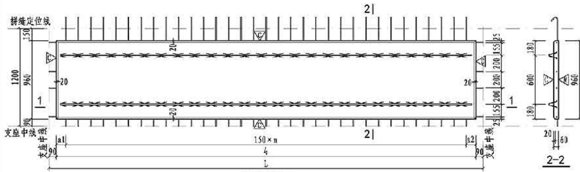
板模板图
