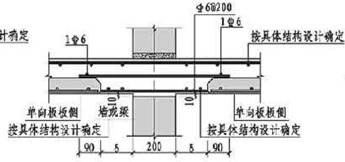
中间支座构造(三)
