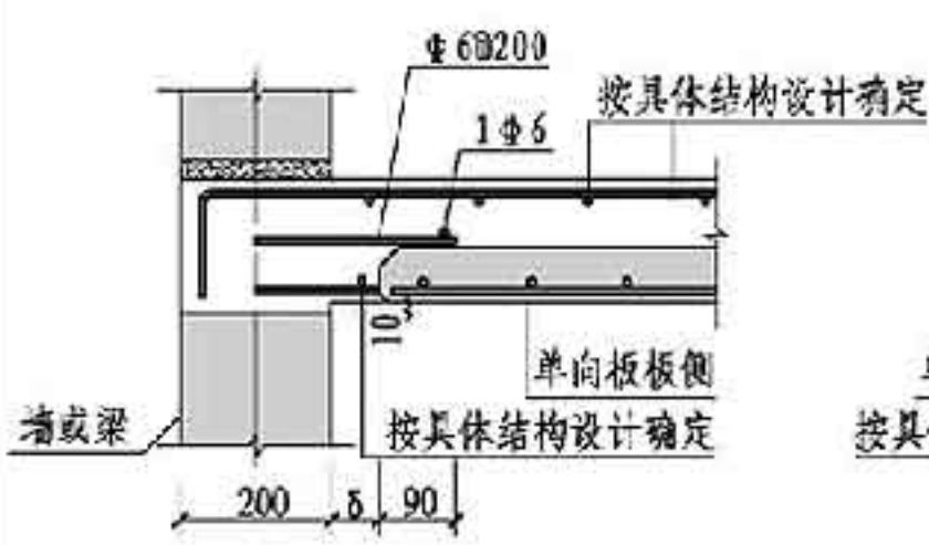
侧支座构造(二)
