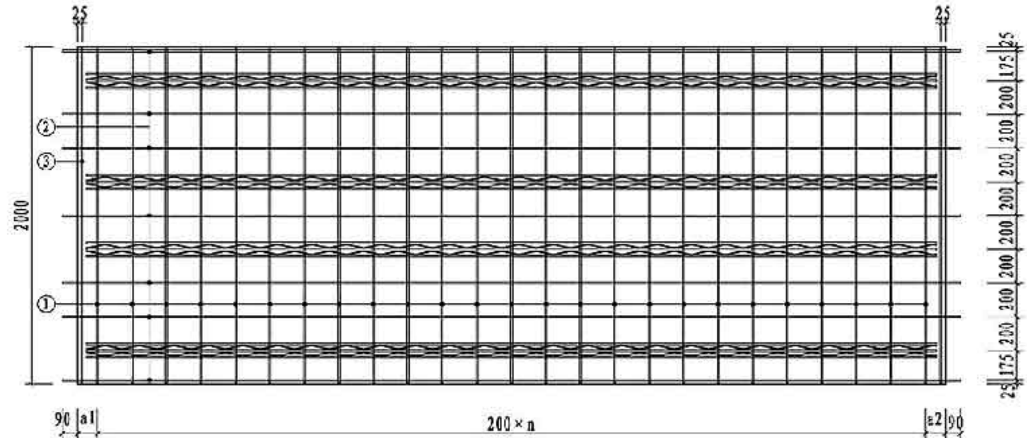
板配筋图
