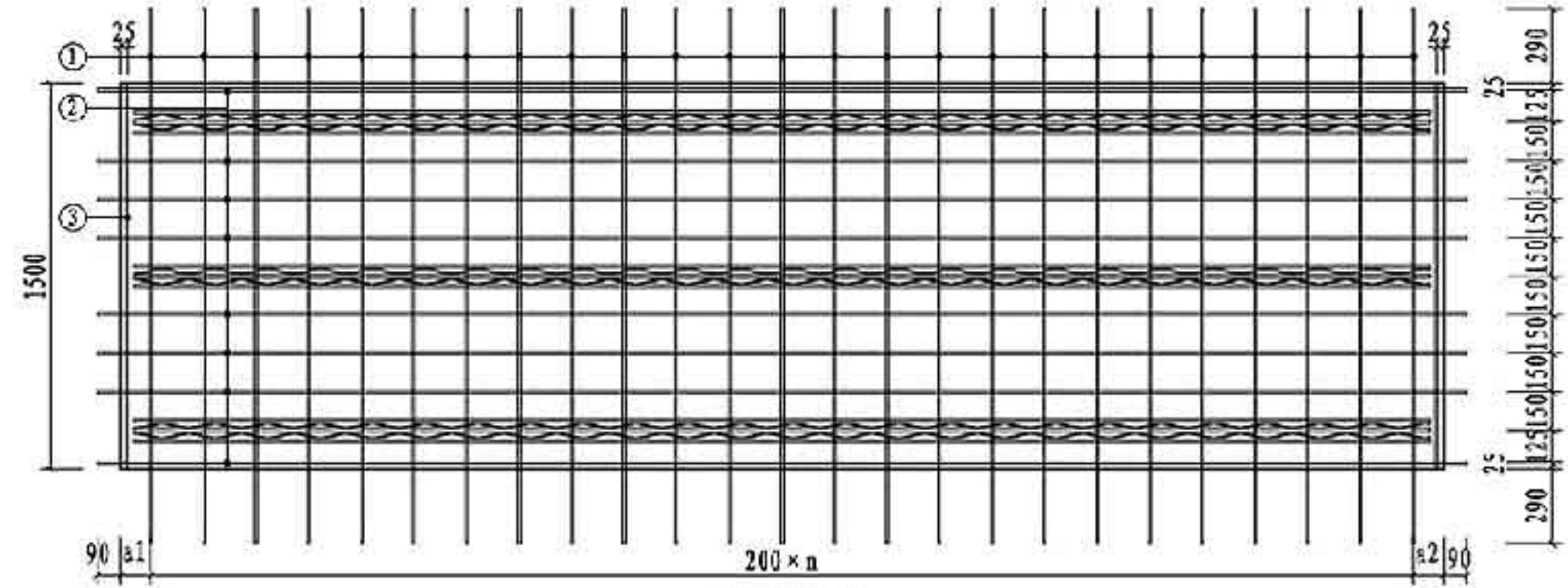
板配筋图
