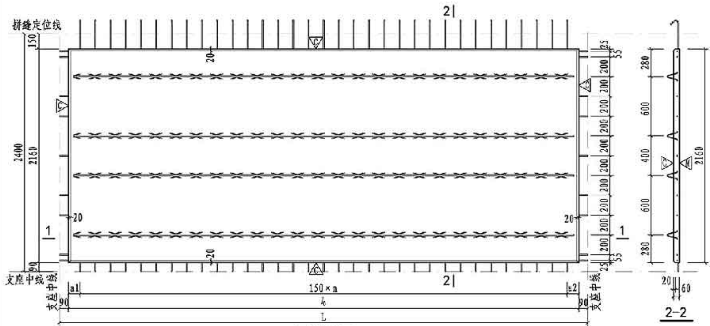
板模板图
