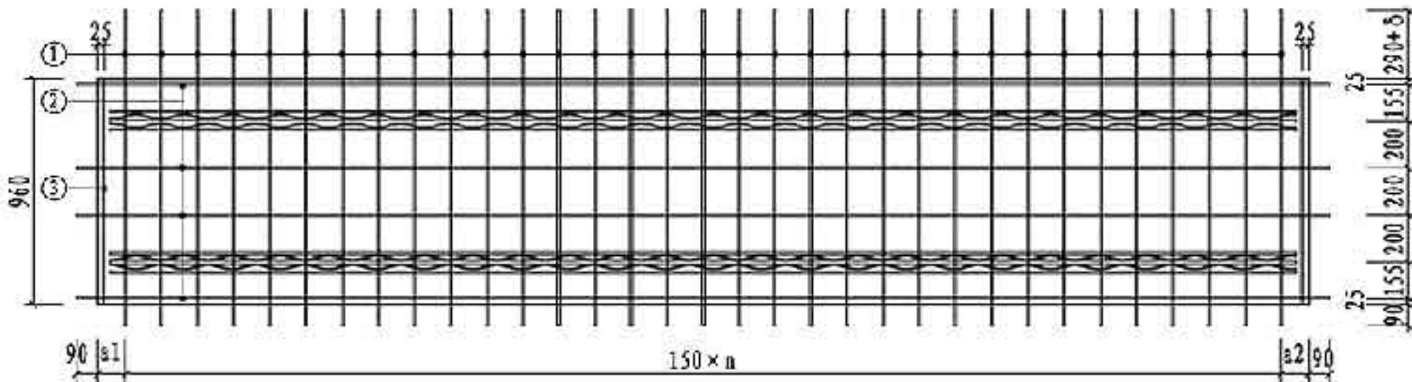
板配筋图
