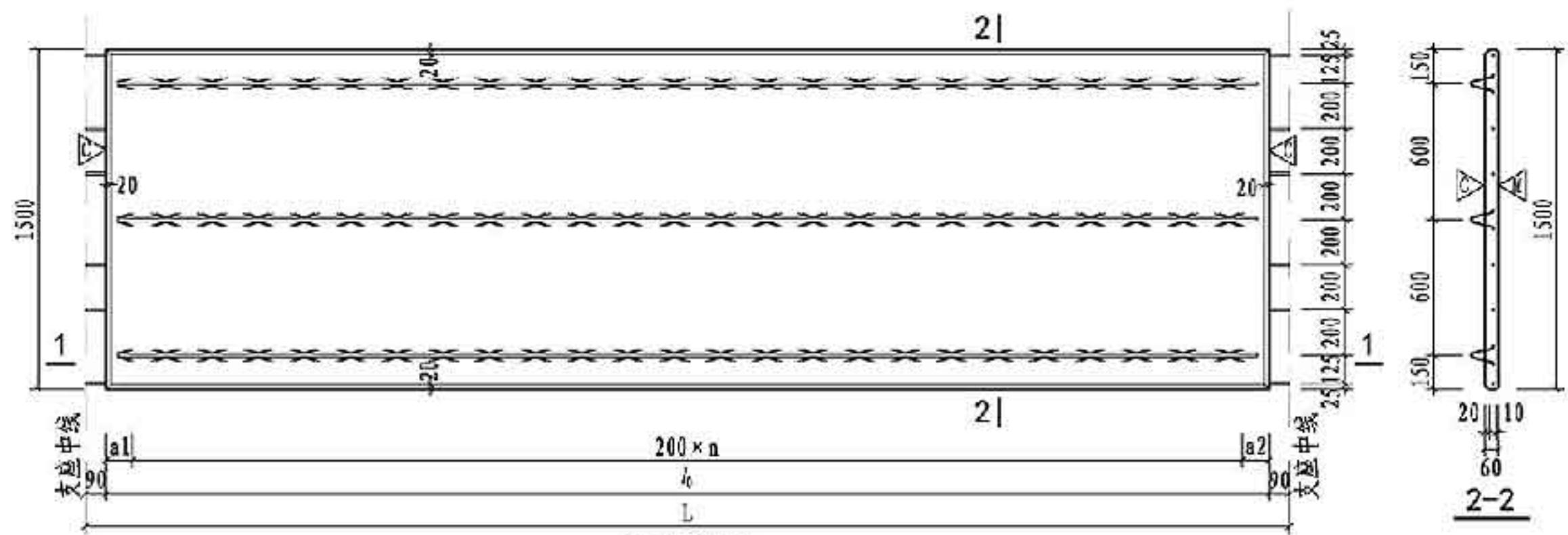
板模板图
