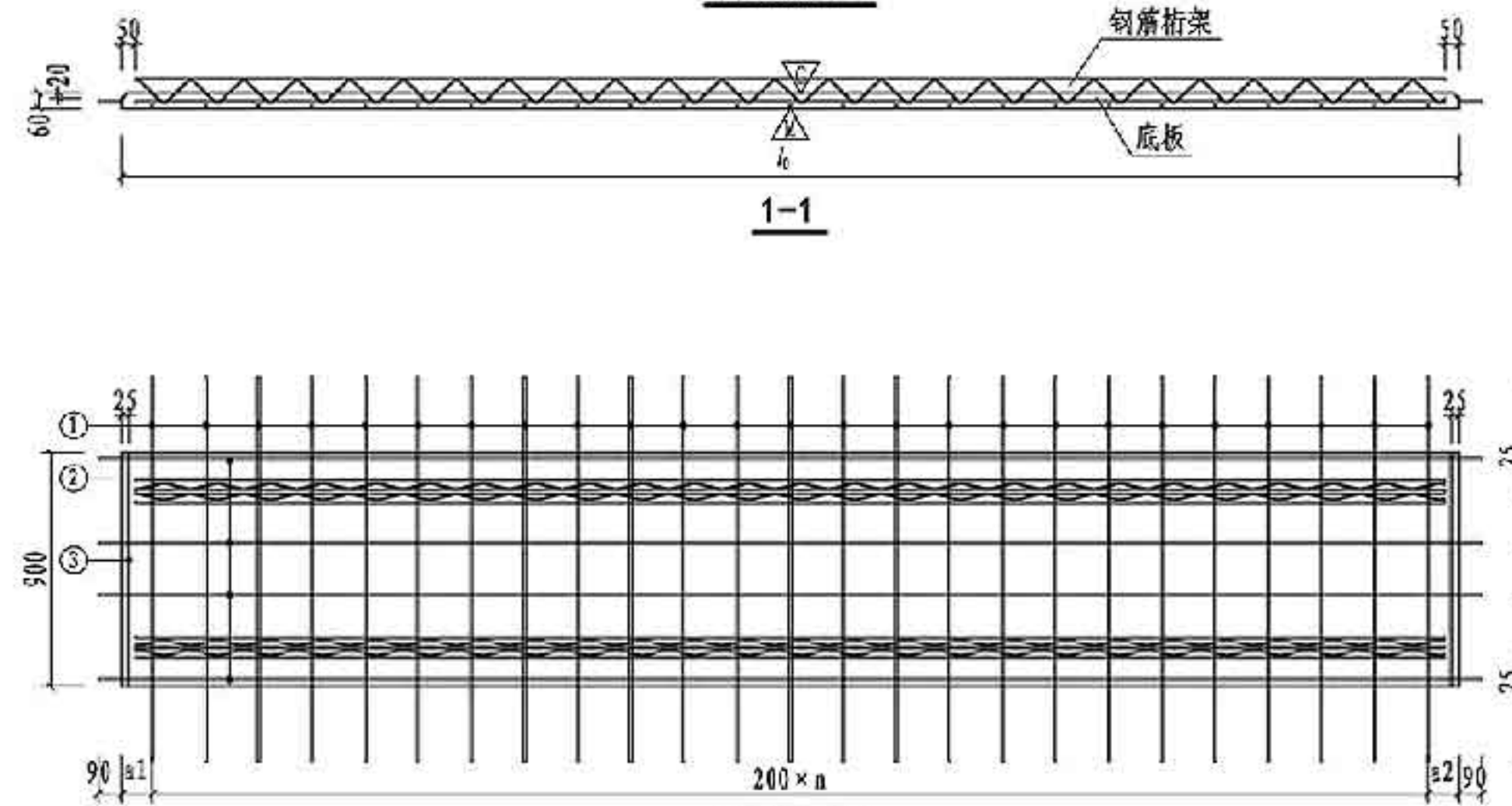
板配筋图
