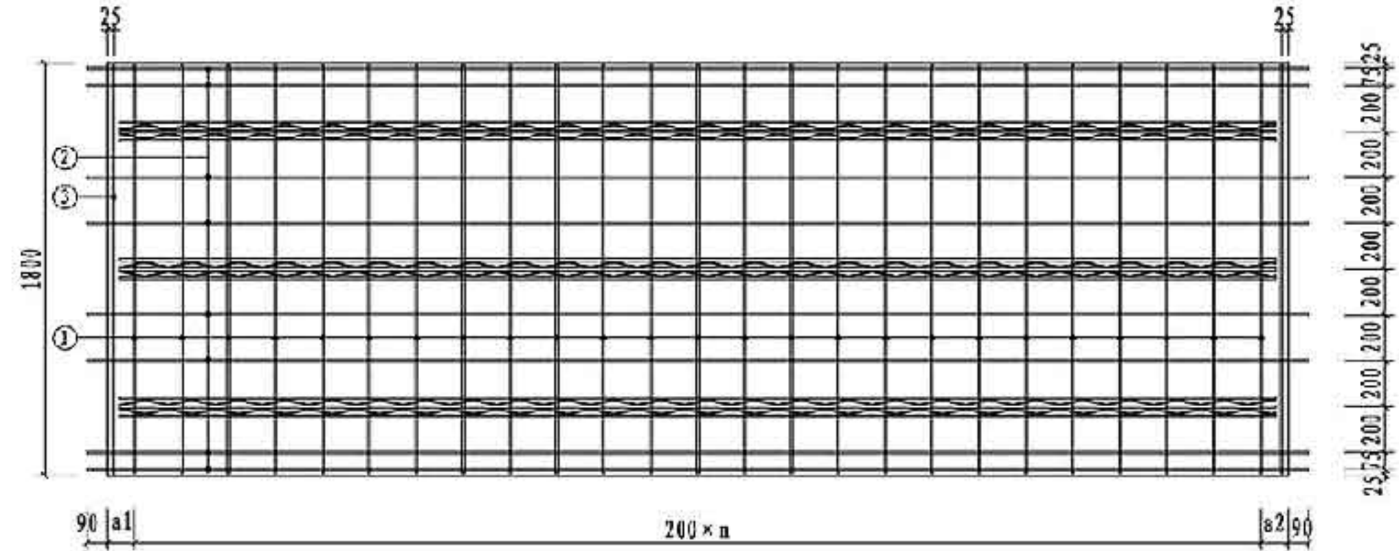
板配筋图
