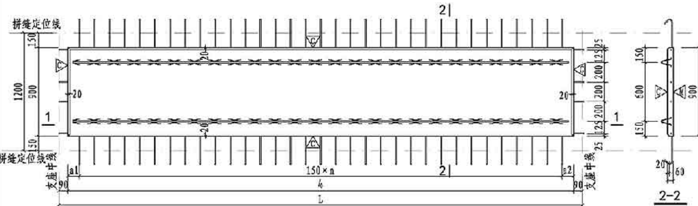
板模板图
