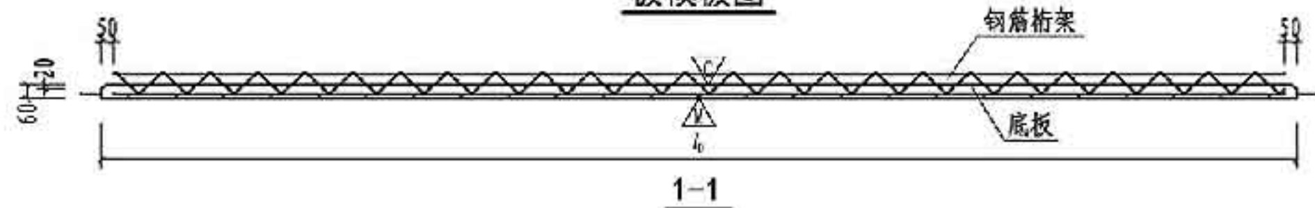
板模板图
