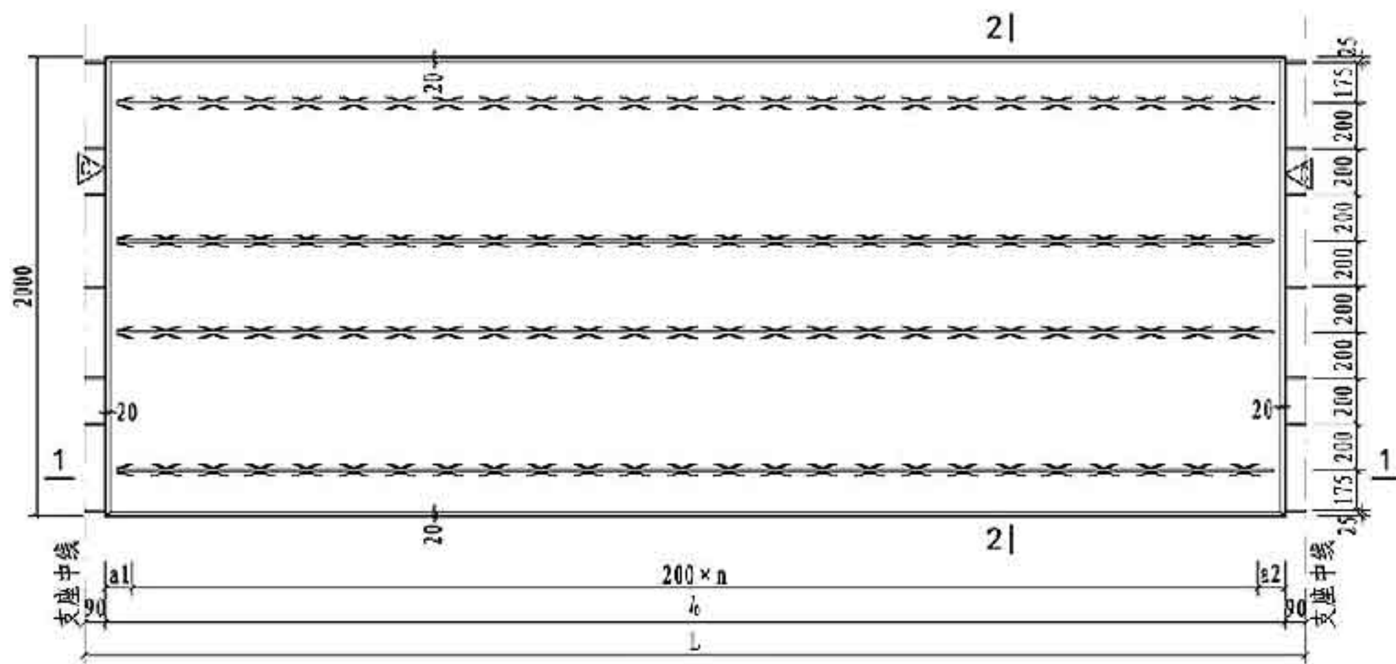
板模板图
