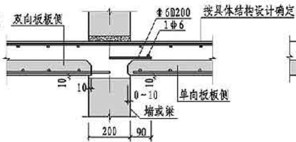
中间支座构造(七)
