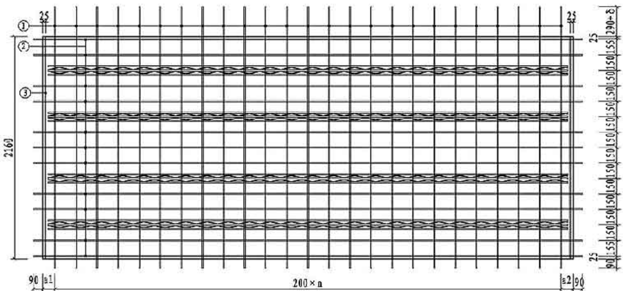
板配筋图
