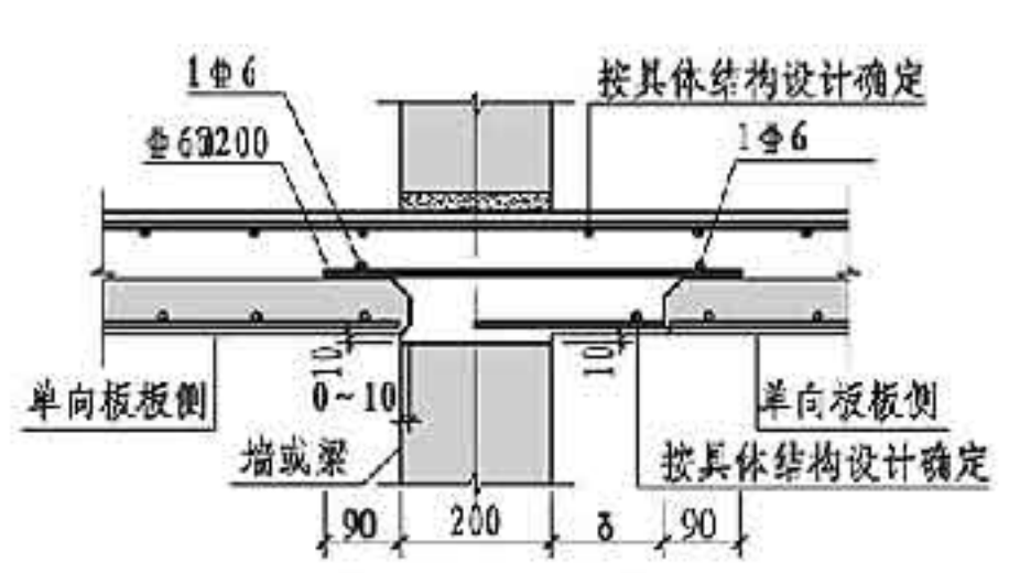
中间支座构造(九)
