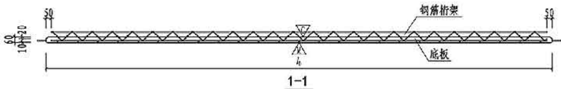
板模板图
